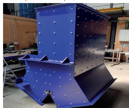
Fabrication d'une trémie.
